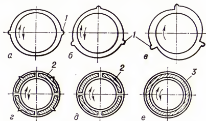
Рис. 2. Схемы радиальных подшипников скольжения высокоскоростных роторов: а — эллиптический; а, б — с жёсткими секторами; в — из смешанных секторов; г — из секторов, образованных качающимися вкладышами; д — из свободных вкладышей; е — с «плавающим» вкладышем; 1 — место подвода смазки; 2 — сектор; 3 — кольцеобразный «плавающий» вкладыш.
